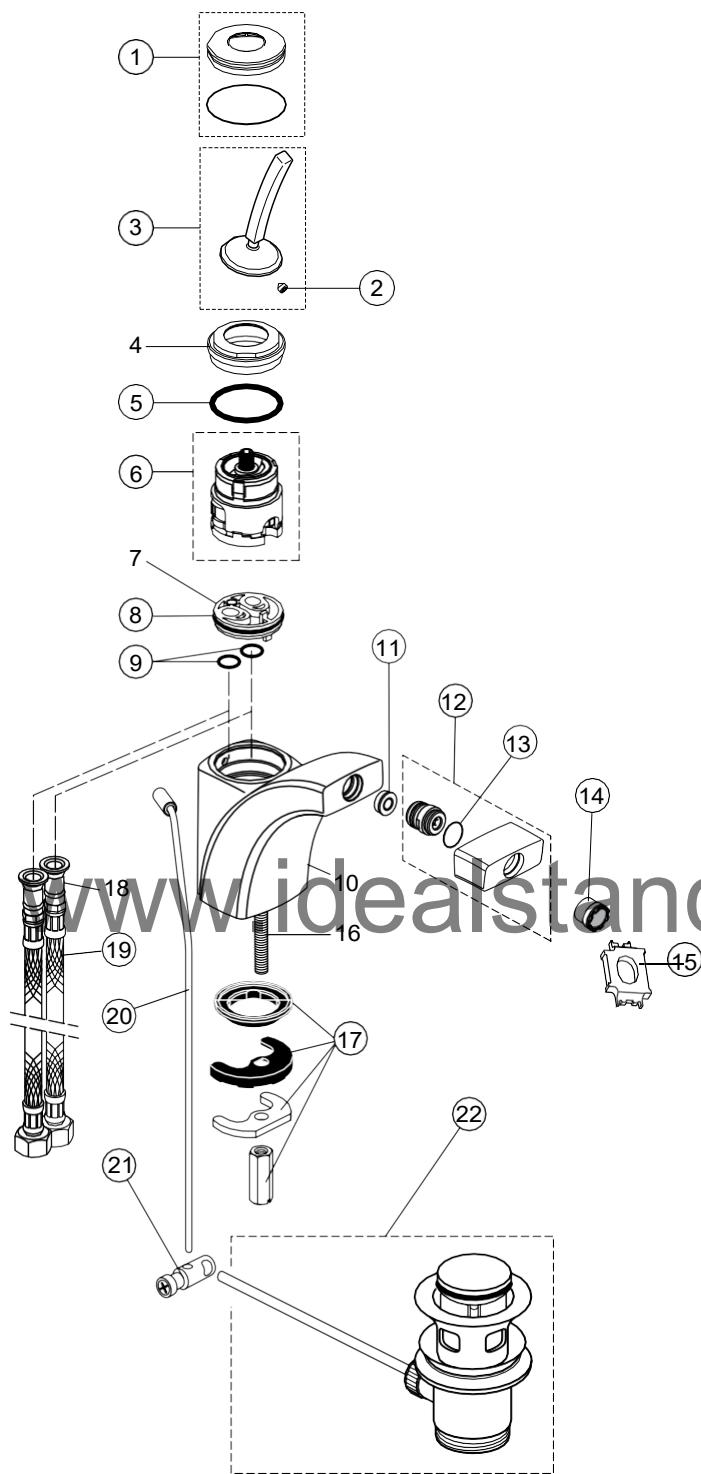
1-Loch Bidetbatterie chrom, mit Ab- und Überlaufgarnitur AKUA A4035AA
