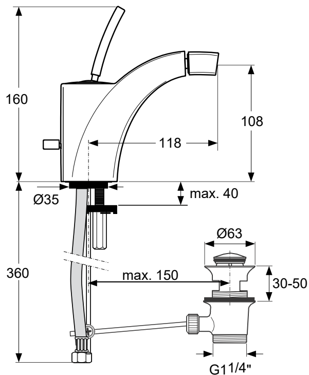
1-Loch Bidetbatterie chrom, mit Ab- und Überlaufgarnitur AKUA A4035AA
